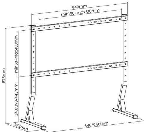
Abmessungen
