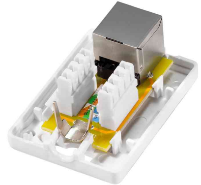
Anschlussdose Kat.6A mit Aufputzbox, 1 x RJ45
